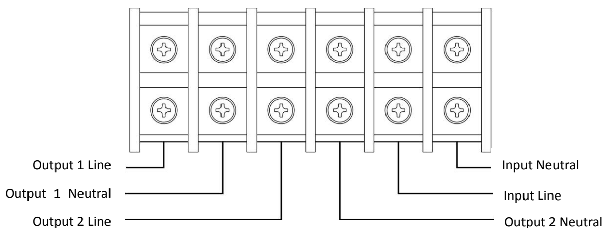
Schema del terminale 6000(L)/10000(L)
