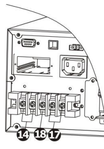
Figura 4: Terminali entrata/uscita
