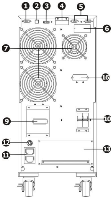
Şekil 1: 6000(L)/10000(L) Arka Panel Görünüşü
