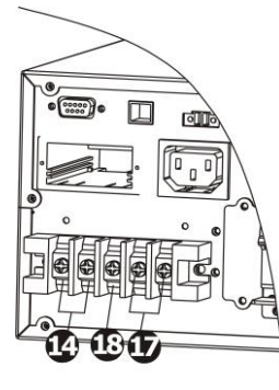
Figura 4: Terminales entrada/salida
