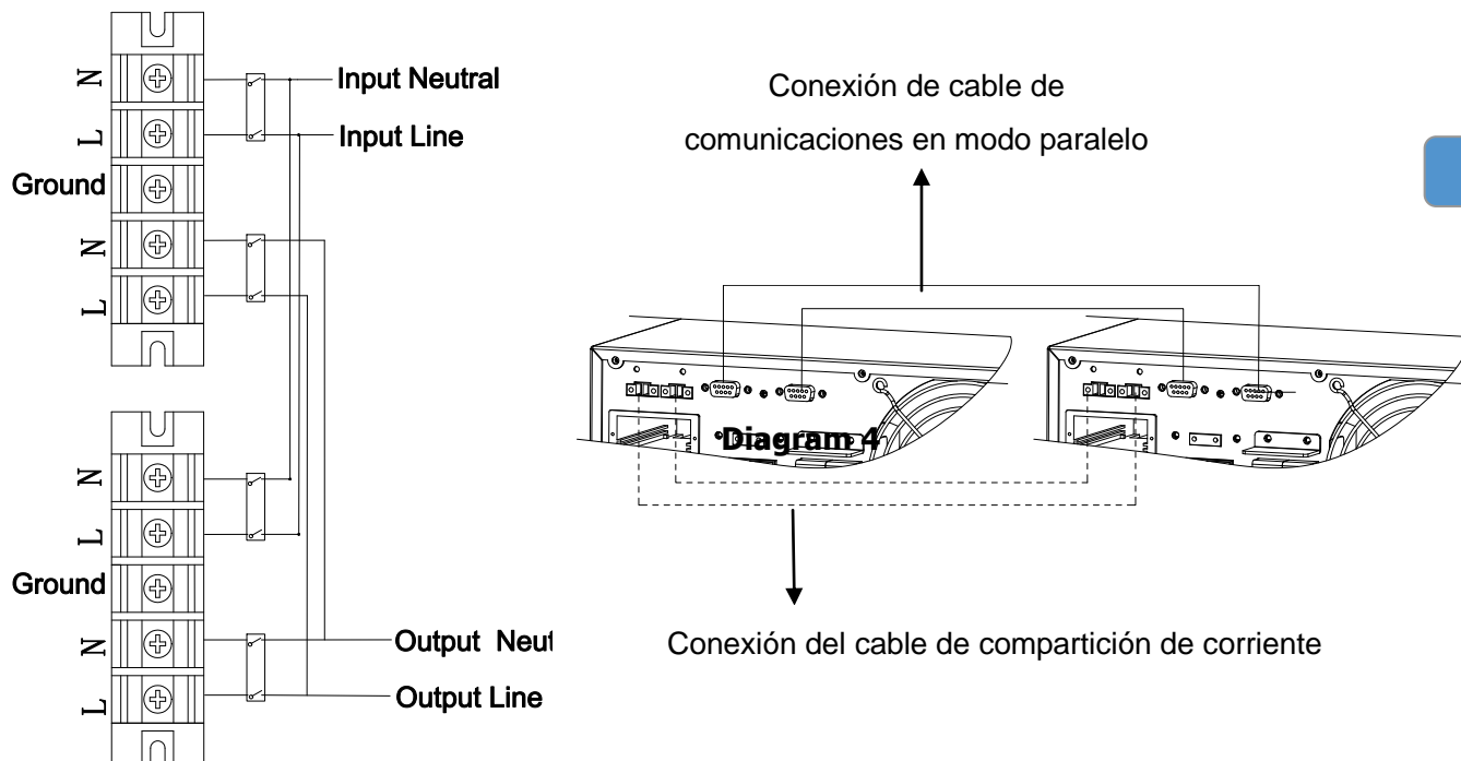
Figura 1: Esquema de conexión
