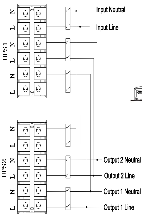
Diagrama 1: Ligação do cabo de alimentação
